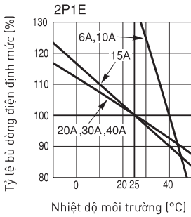
Đường cân bù nhiệt độ
