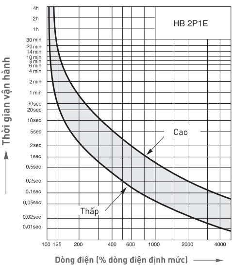
Đường cong đặc tính vận hành
