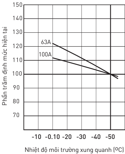
Đồ thị bù theo môi trường xung quanh
