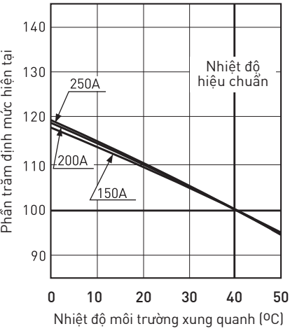
Đồ thị bù theo môi trường xung quanh
